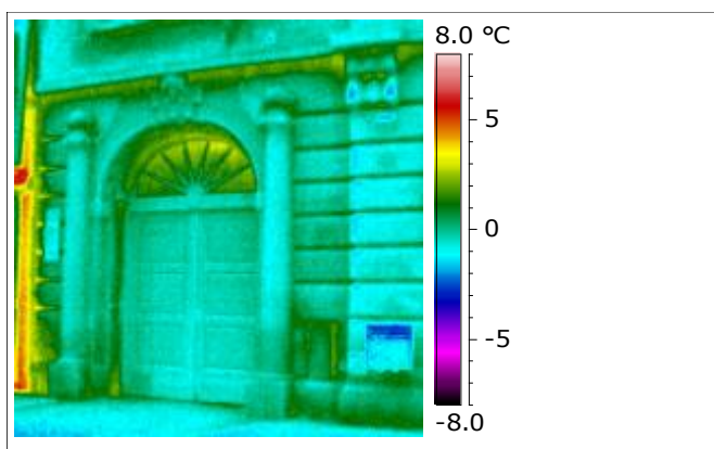
Jižní pohled (dvůr)
