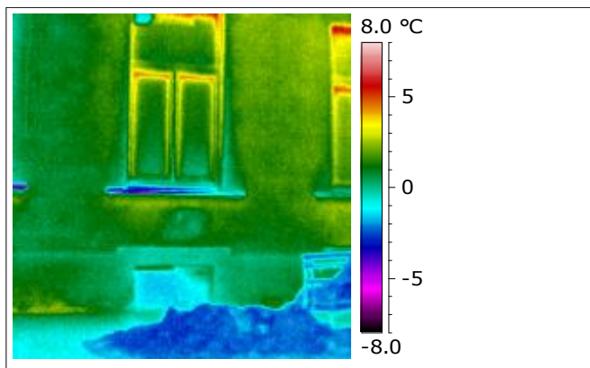
Severní pohled (dvůr)
